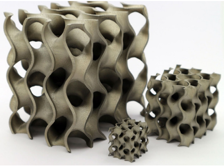
Laser Beam Melting (LBM): Gyroidstruktur mit Edelstahllegierung
